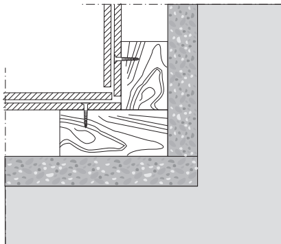
10. Binnenhoekoplossing zonder profiel
