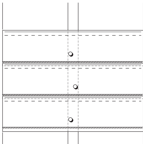
tekening B: verspringen van nagels / schroeven ter voorkoming van scheuren/splijten regelwerk
